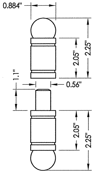
9 HINGE
